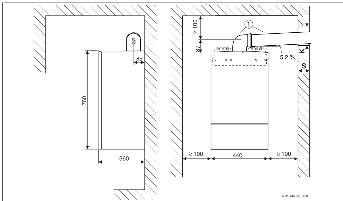
Fig. 6 Conducción de gases Ø 60/100 mm
