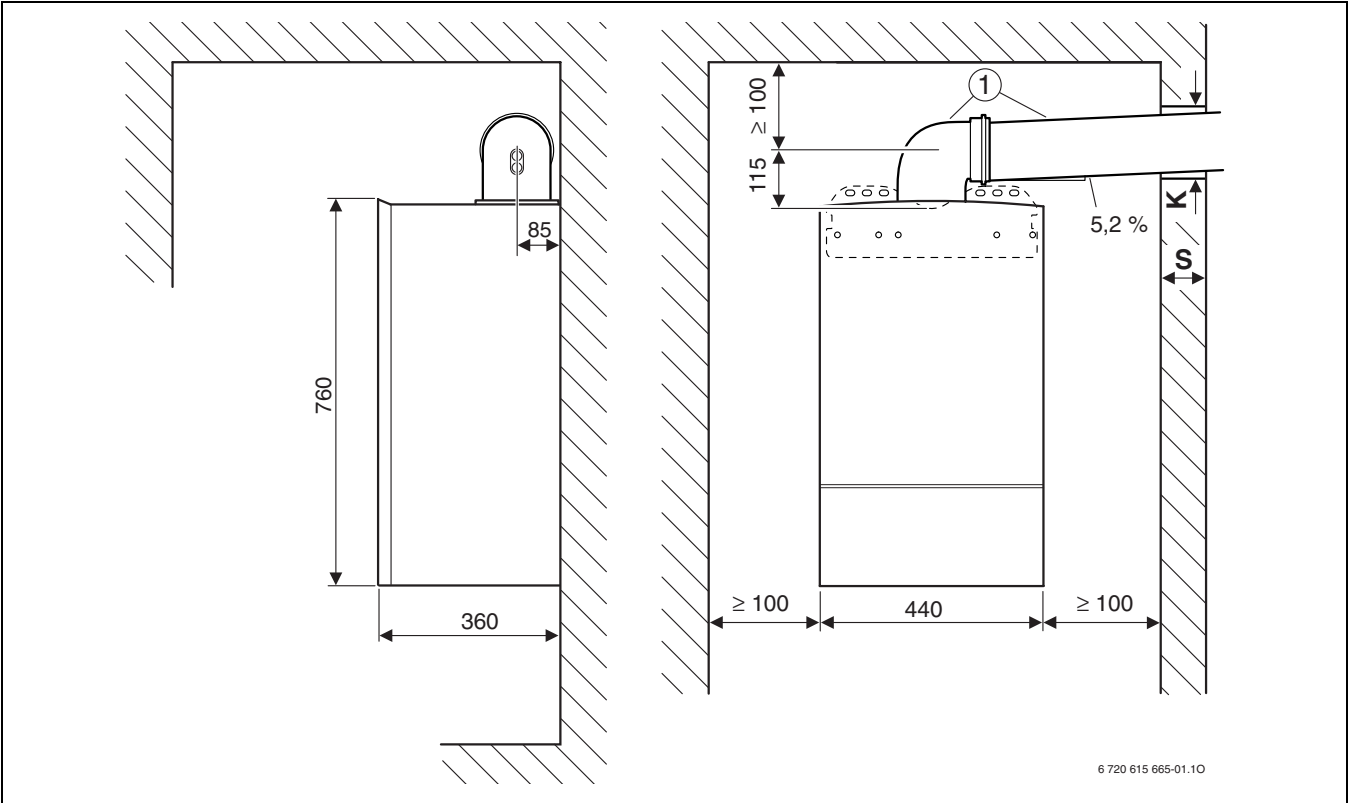
Fig. 5 Conducción de gases Ø 80/125 mm o Ø 80 mm
